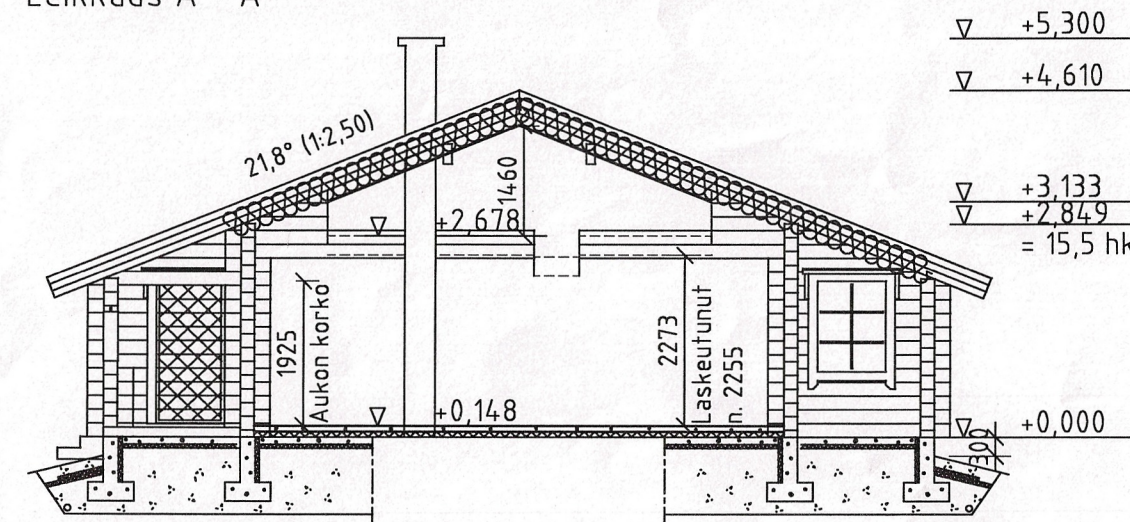
PERUSTUKSET JA SALAOJITUKSET ERIKOISSUUNNITELMIEN MUKAAN
