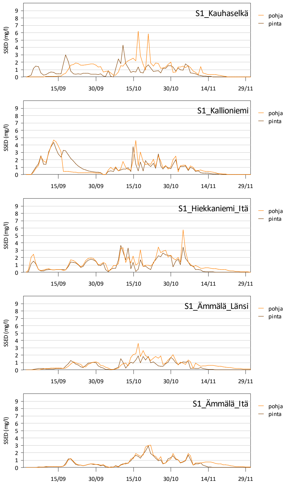
Kuva 7: Ruoppauksen aiheuttama kiintoainepitoisuuden nousu Kauhaselän eri pisteissä (vuorokauden keskipitoisuus).
