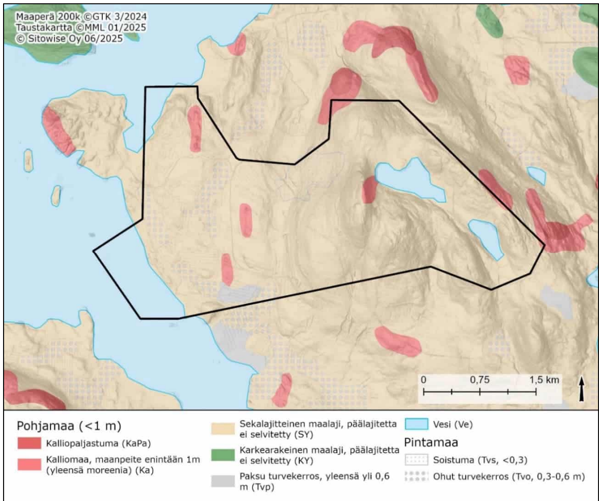
Kuva 5.2. Kaava-alueen maaperä. Kaavaraja mustalla.
