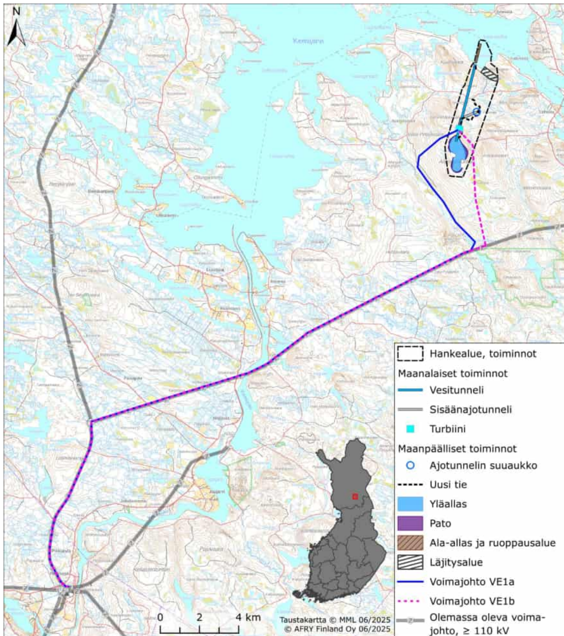
Kuva 1-1. Hankealueen sijainti ja raja- seuraavassa kuvassa (Kuva 1-1). Hankkeeseen kuuluu allasalue Ailangan- tunturilla ja voimajohto Pirttikosken sähköasemalle.
