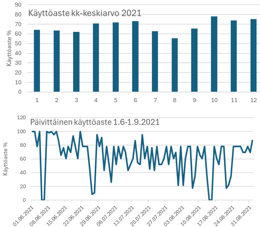
Kuva 4-1. Pumppuvoimalan käyttöasteen, ts. päivittäisen ulosvirtaaman osuus yläaltaan tilavuudesta (%), kuukausikeskiarvot vuonna 2021 ja päiväarvot kesälle 2021.
