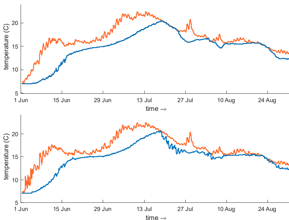
Kuva 8-1. Pinta- ja pohjakerroksen lämpötilan aikasarja Kauhaselän pisteessä, nykytila ylemmässä kuvassa, pumppuvoimalan kanssa alemmassa kuvassa. Pisteiden syvyys noin 15 m. Oranssi käyrä pintakerros, sininen käyrä pohjakerros.
