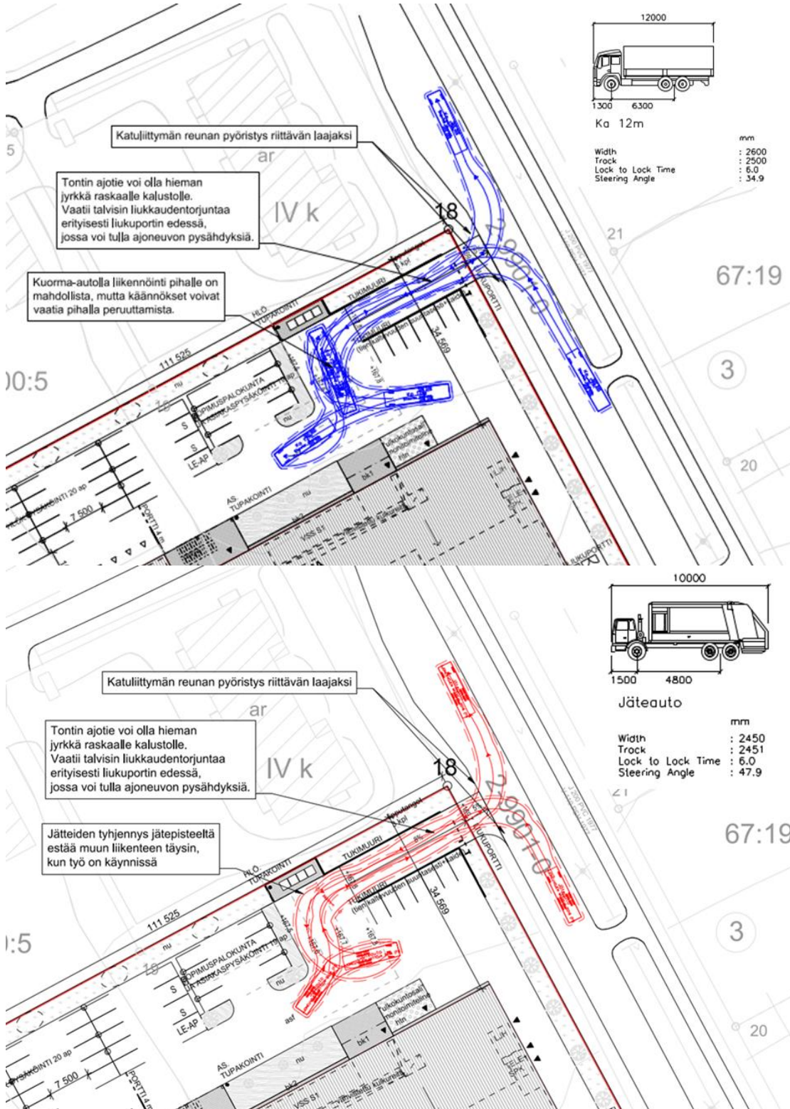
Kuva 6. Huoltoliikenteen ajourat.
